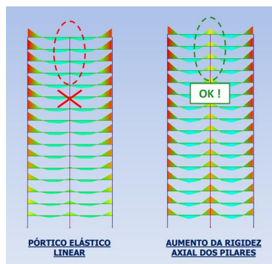
Figura 5 – Configurações de dimensionamento: a) Configurações de análise; b) Consideração do aumento da rigidez axial dos pilares
